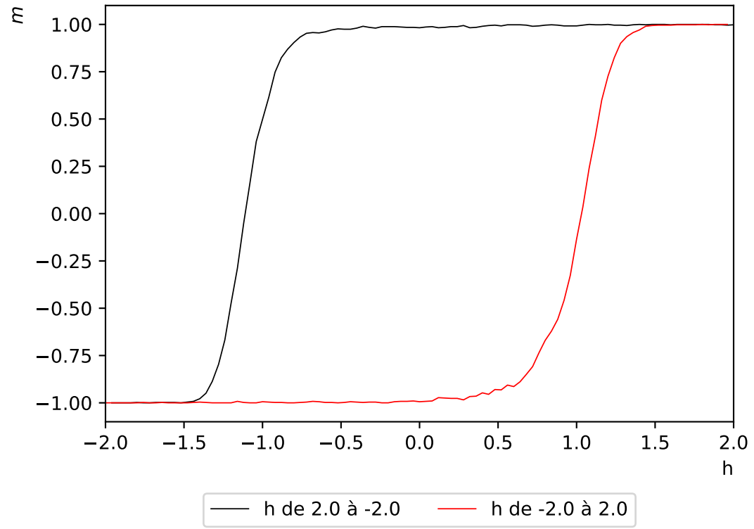
Hystérésis de l'aimantation - réseau de taille L=32 - champ magnétique d'amplitude h=2 à T=1.5
